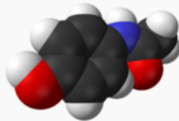
Représentations plane et 3D d'une molécule de paracétamol
